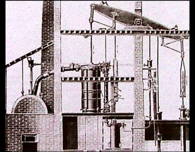
Паровий двигун обертання Дж. Уатта. Англія. 1788.
